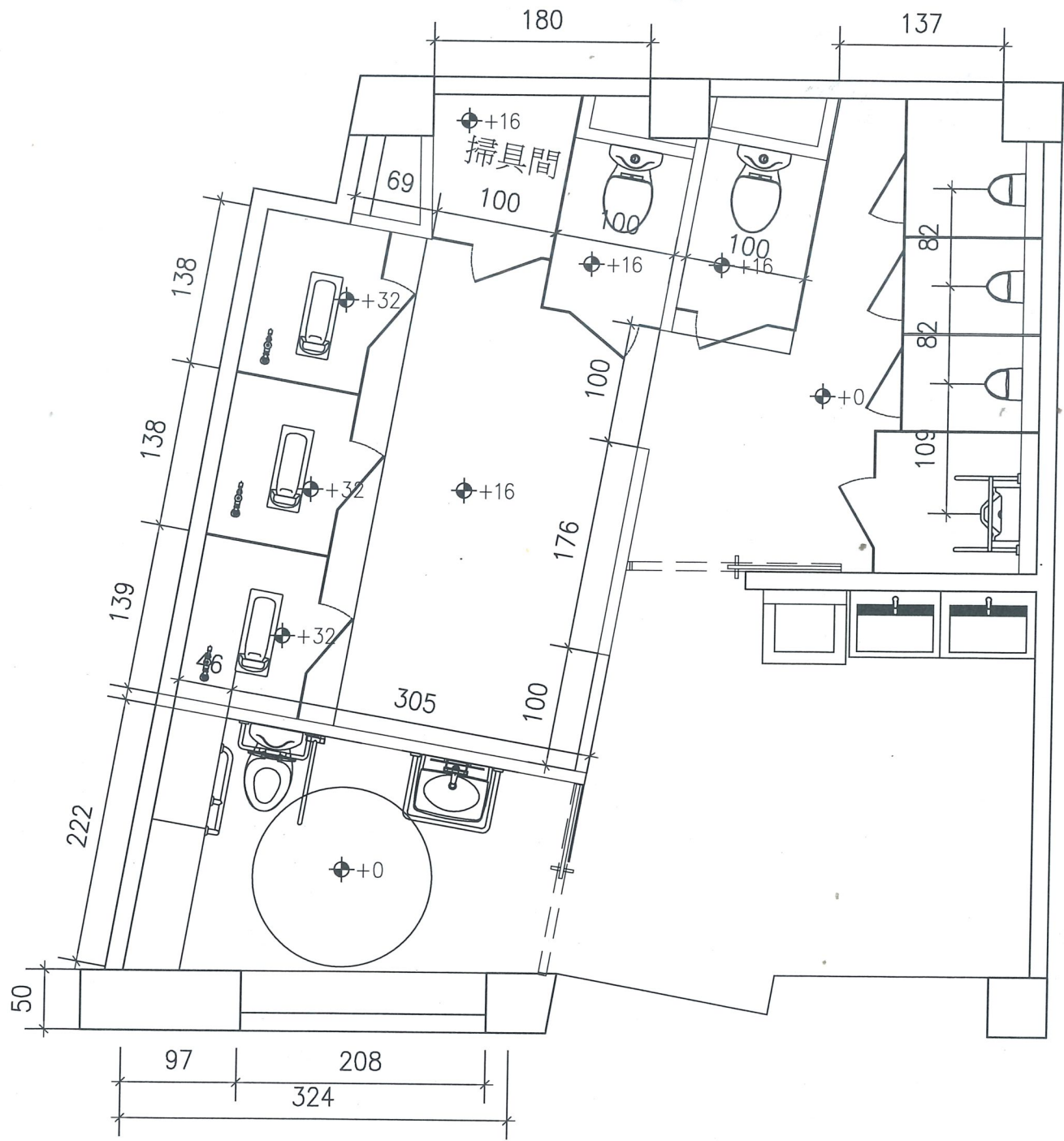
二樓性別友善廁所設計平面
